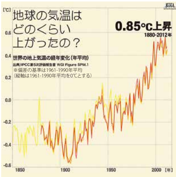
【図2】世界の地上気温の経年変化(年平均)
